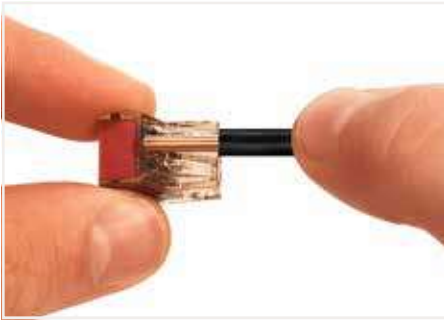
剝去單芯導線絕緣外皮 12 mm (0.47 inch)。
