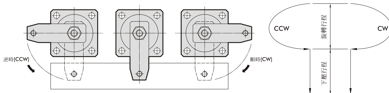
雙邊壓板旋轉示意圖
